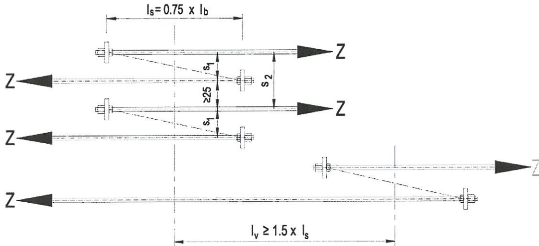
Bild 2: Beispiel für die Stoßausbildung nach Abschnitt 4.1.4
