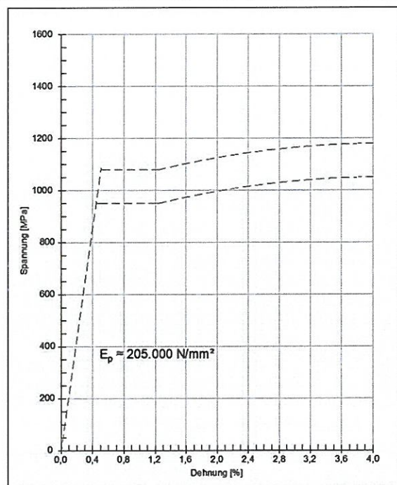
Bild 2: Prinzipieller Spannungs-Dehnungsverlauf
