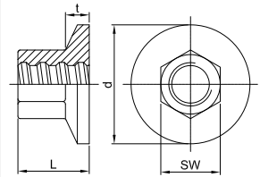
Ankerstück anchor piece
